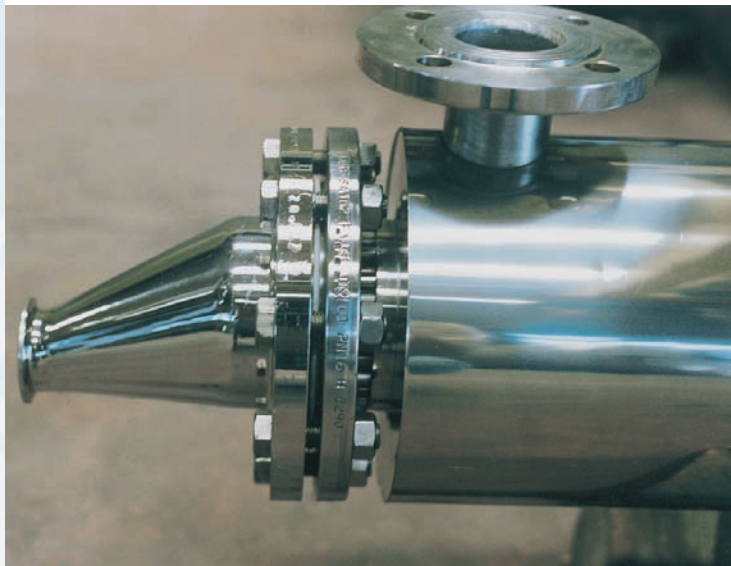
Particolare testata a passaggio unico Detail head single passage
