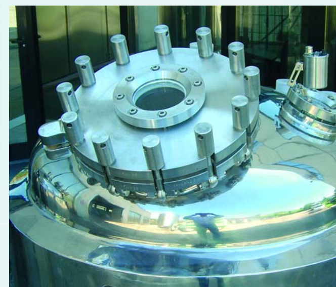
▲ Particolare passo d'uomo con specula visiva Detail of man hole with sight glass
